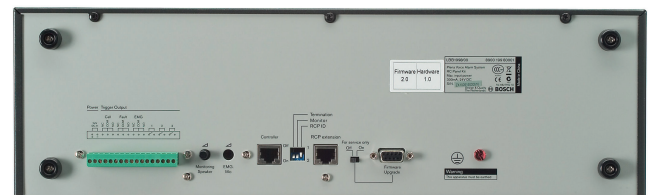
LBB 1998/00 后视图
